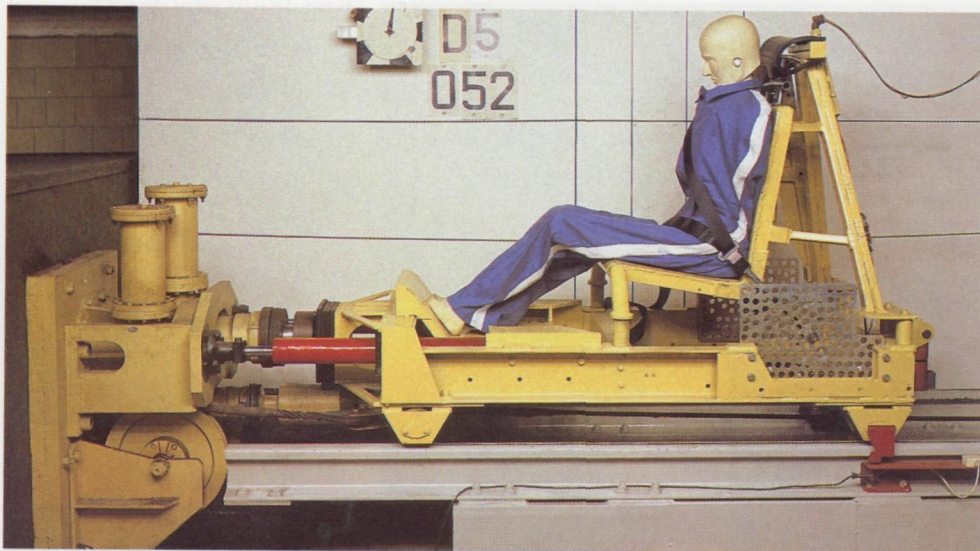
Ohutusrihmade dünaamilise katse stend
