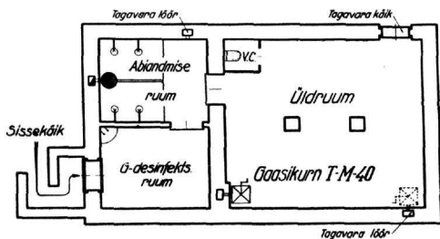
G-kurna asetusvõimalusi varjendis
