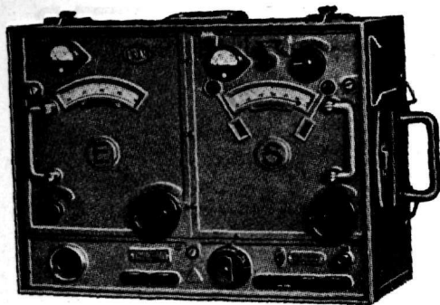
Ühevatilise võimsusega väliraadiojaam, mis koosneb saatjast ja vastuvõtjast
