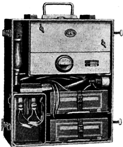
Väliraadiojaama vooluallikad. Ülal käsigeneraator, all anoodpatareid ja aku
