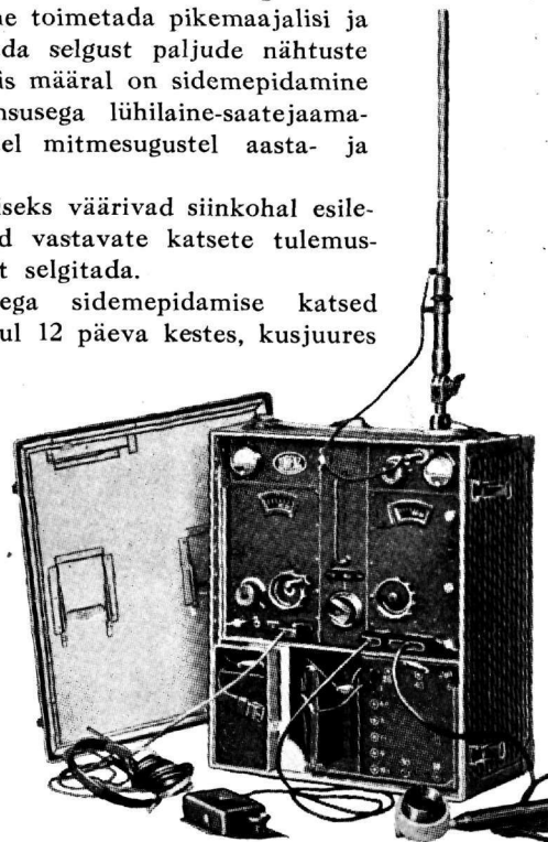
Ühe mehe poolt kantav väliraadiojaam
