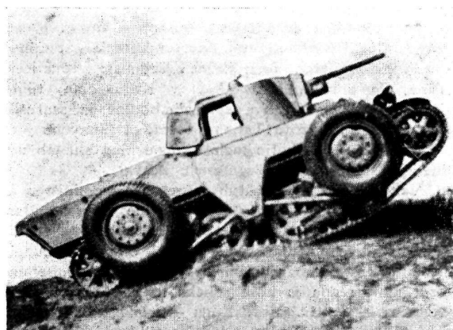
Rootsi lülikratatank
