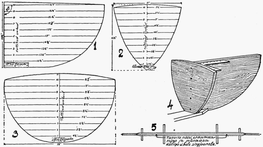
1. Nina ja päraosa. 2. Otsapoolne umbribi. 3. Keskmised umbribid. 4. Ninaosa koos umbribi ja kiiluga. 5. Eelnimetatud osad kokkupandult, altvaates.
