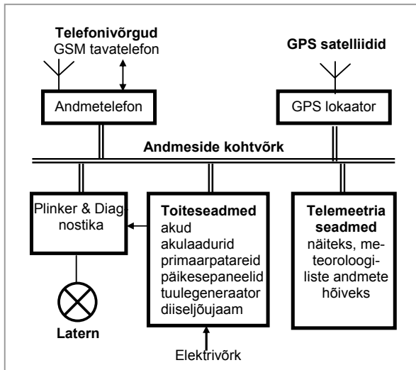
Joonis 1. Tulemärgi automaatikasüsteem.
