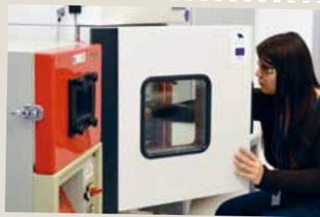
Pildil on kliimakapp, mis võimaldab katsetada kosmosetehnikat näiteks õhutemperatuuril -40...+150 °C ja õhuniiskusega kuni 90%.
