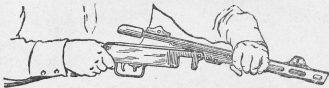
Рис. 38. Как отделить ствольную коробку от затворной
