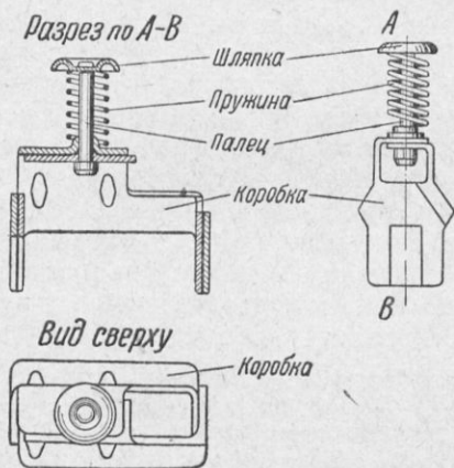
Рис. 58. Приспособление для снаряжения коробчатого магазина
