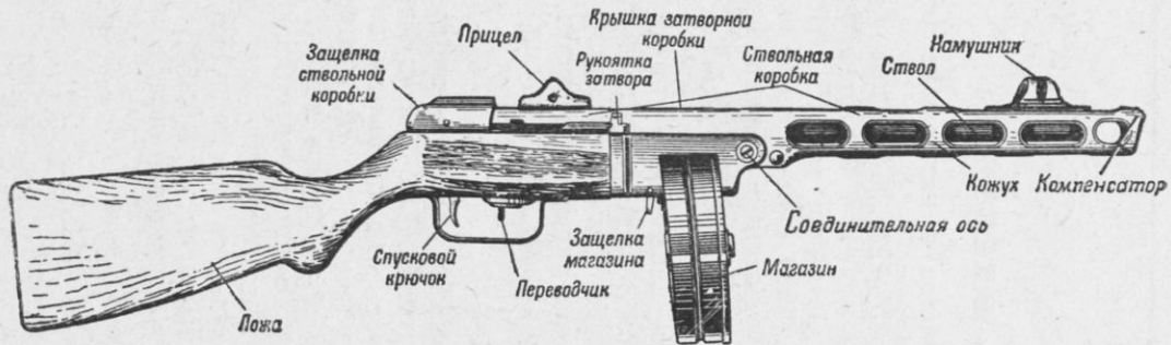
Рис. 1. Общий вид автомата обр. 1941 г. (с дисковым магазином)
