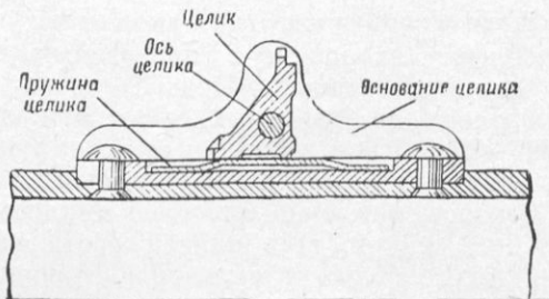
Рис. 6. Прицел с вращающимся целиком
