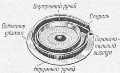
Рис. 23. Улитка
