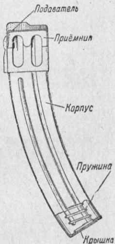
Рис. 27. Коробчатый магазин
