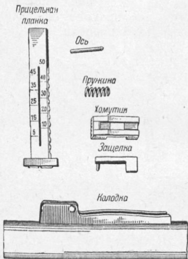
Рис. 7. Секторный прицел
