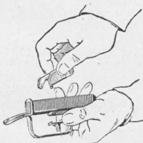
Рис. 47. Как отделить разобщитель с основанием и гнетком от спусковой коробки
