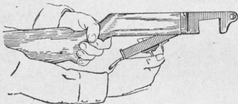
Рис. 42. Как отделить спусковую коробку от ложи
