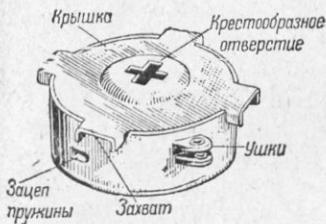
Рис. 24. Барабан
