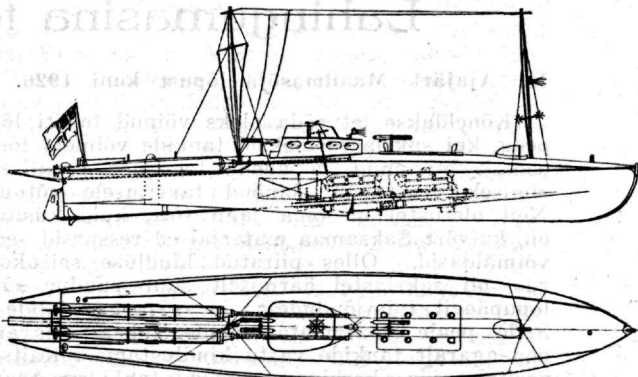
Plaan ja läbilõige kiirmootorpaadist CMB.
