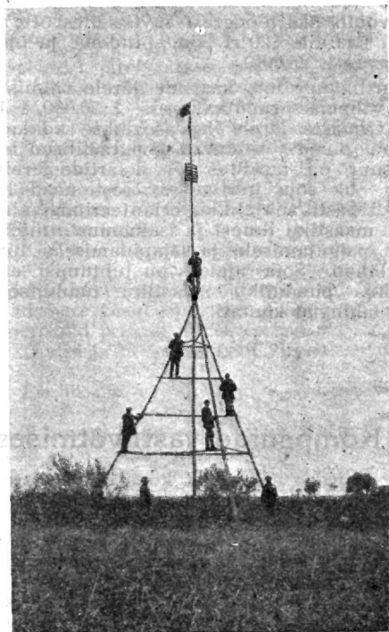
Triangulatsiooni märk Peipsi Sääritsa küla juures.
