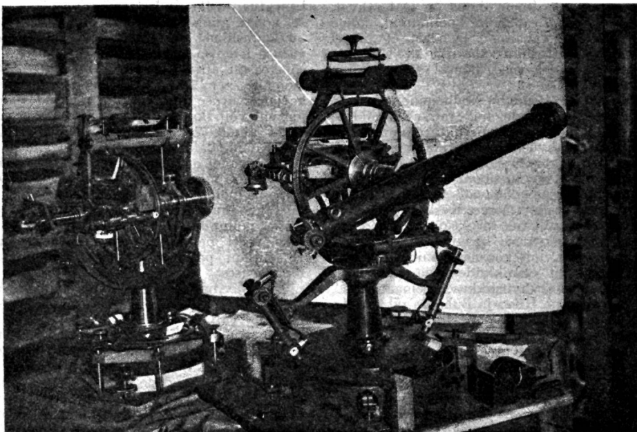
Trianguleerimise juures tarvitatav Hildebrandi universaal-instrument.
