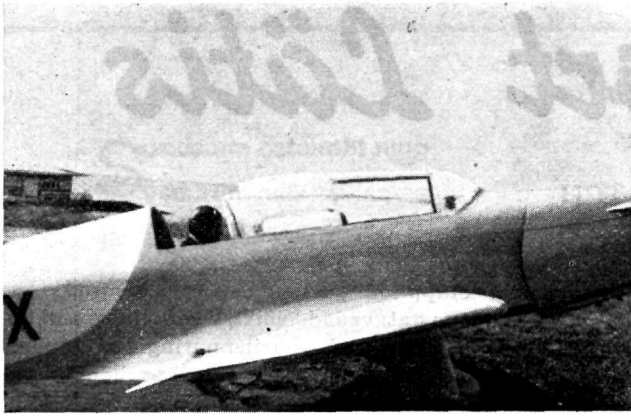
„VEF“ raadiotehaste lennukite osakonnas ehitatud sportlennuk „J 11“ Tallinna lennuväljal
