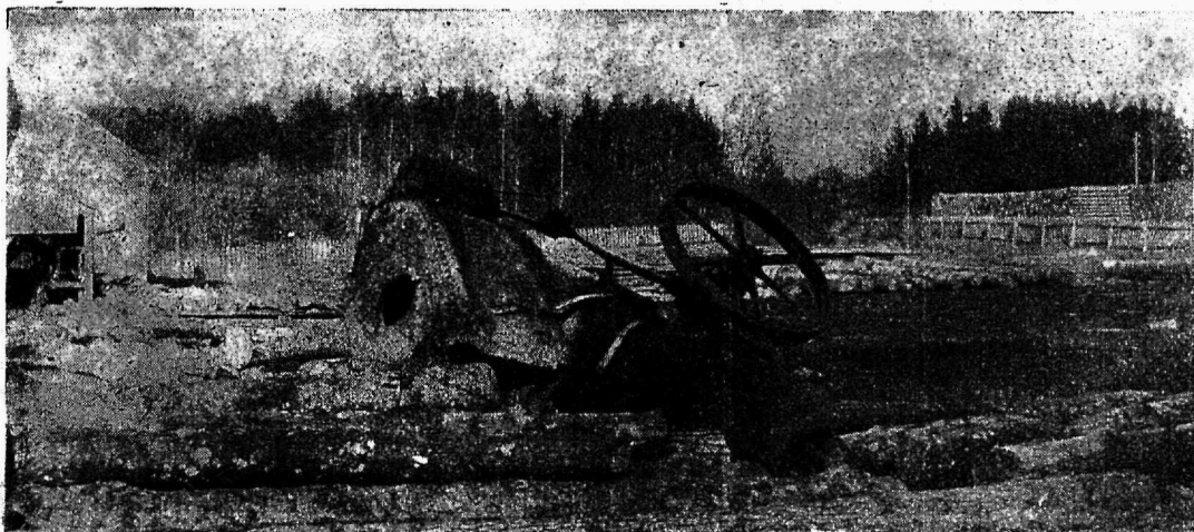
Joon. 4. Lokomobiil peale aurukatla lõhkemist.
