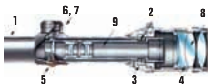
Joonis 6. Sihiku optiline süsteem ( www.milletsights.com ).
