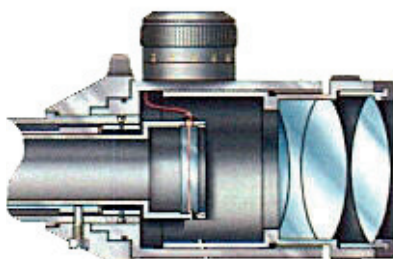
Joonis 7. Okulaar ( www.millettsights.com ).
