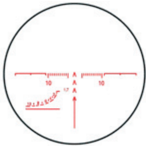
Joonis 10. SVD niitistik. Mõõtskaala inimese kauguse määramiseks on all vasakul.
