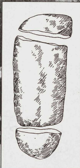
Joonis 3. Nukleus.
