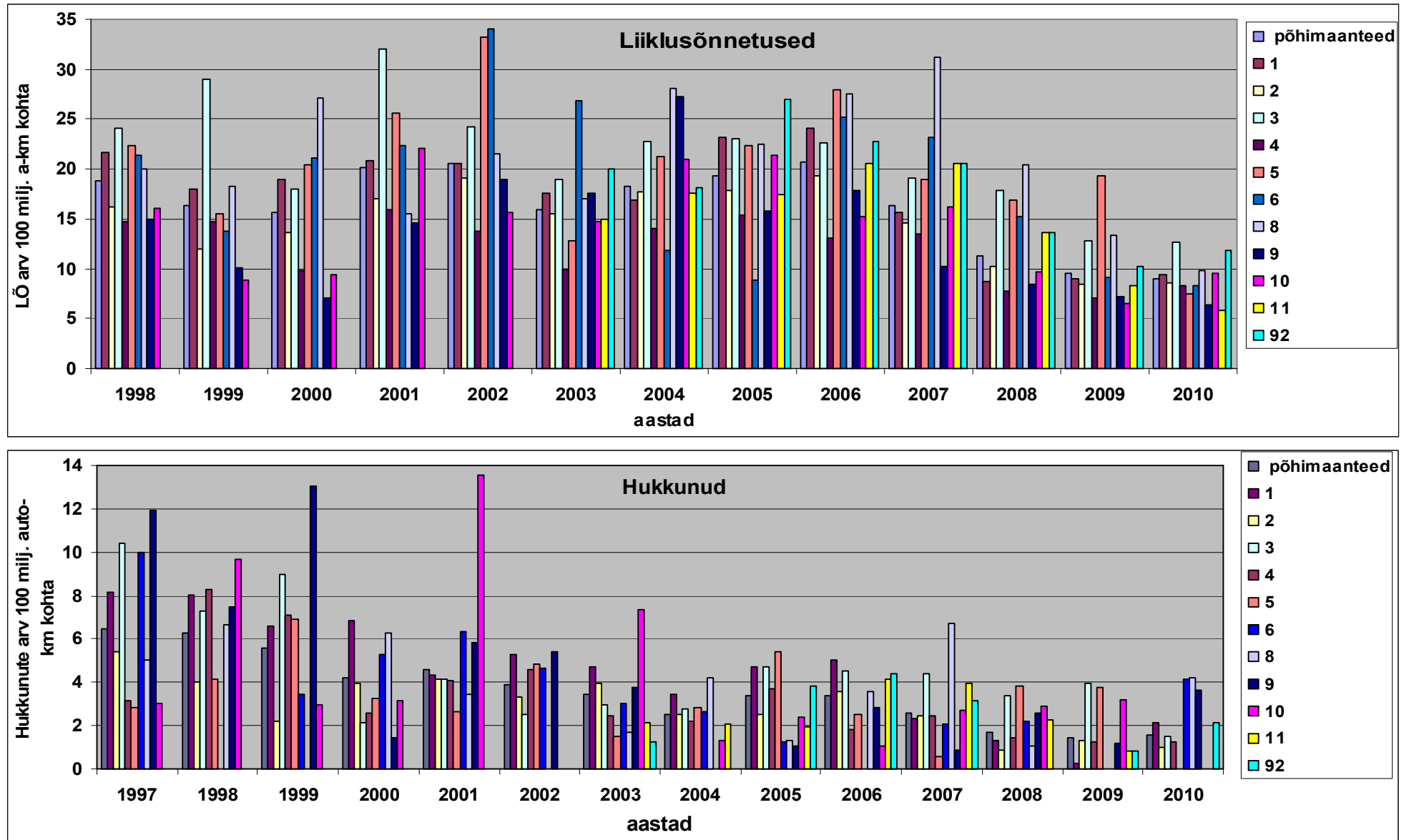
Joonis 3.7 Põhimaanteedel liiklusõnnetuste ja neis hukkunute arv 100 miljoni auto-km kohta aastatel 1997 – 2010. a
