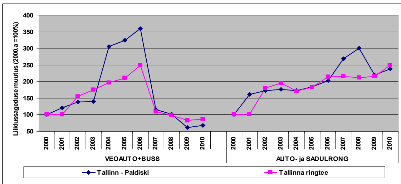
Joonis 1.15 Raskeliikluse keskmise liiklussageduse muutus aastatel 2000 - 2010
