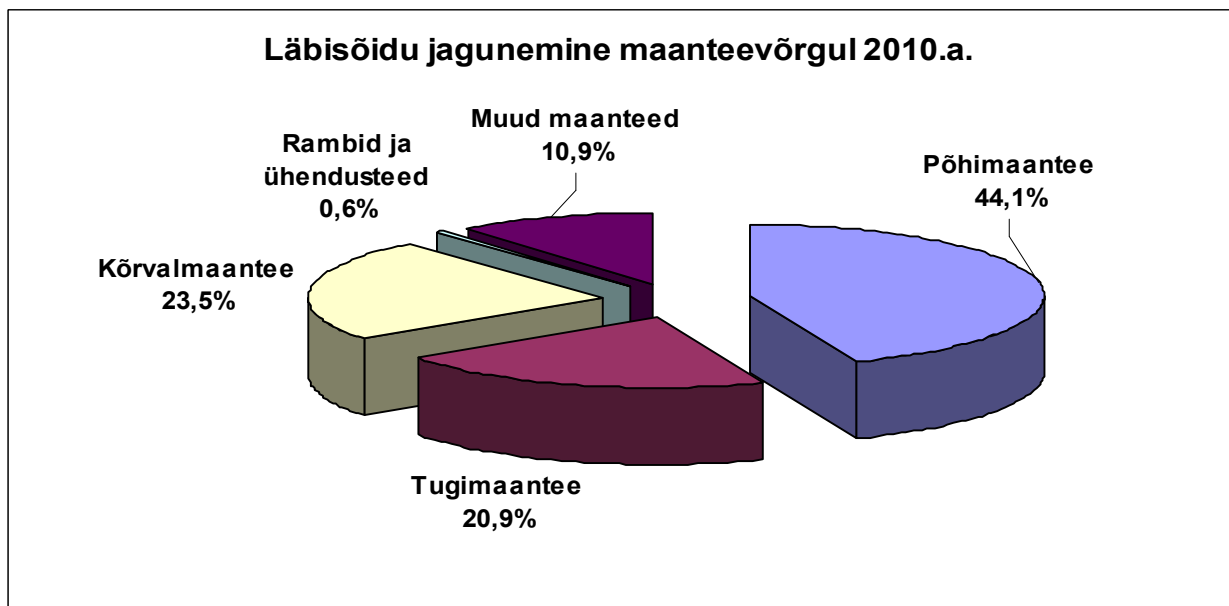
Joonis 1.29 Maanteede liigiline jaotus ja läbisõidu jagunemine maanteevõrgul 2010. aastal
