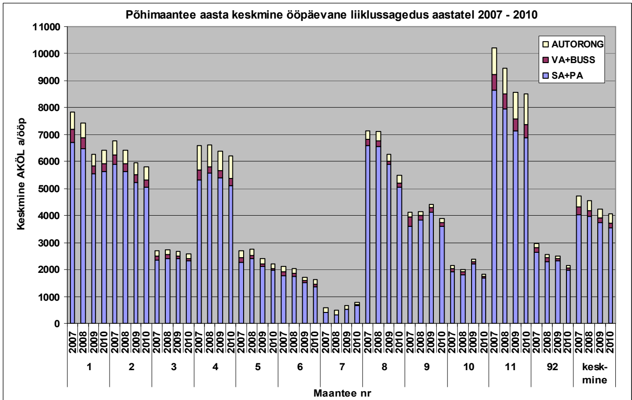
Joonis 1.13 Keskised liiklussagedused põhimaanteedel 2007. kuni 2010. aastal
