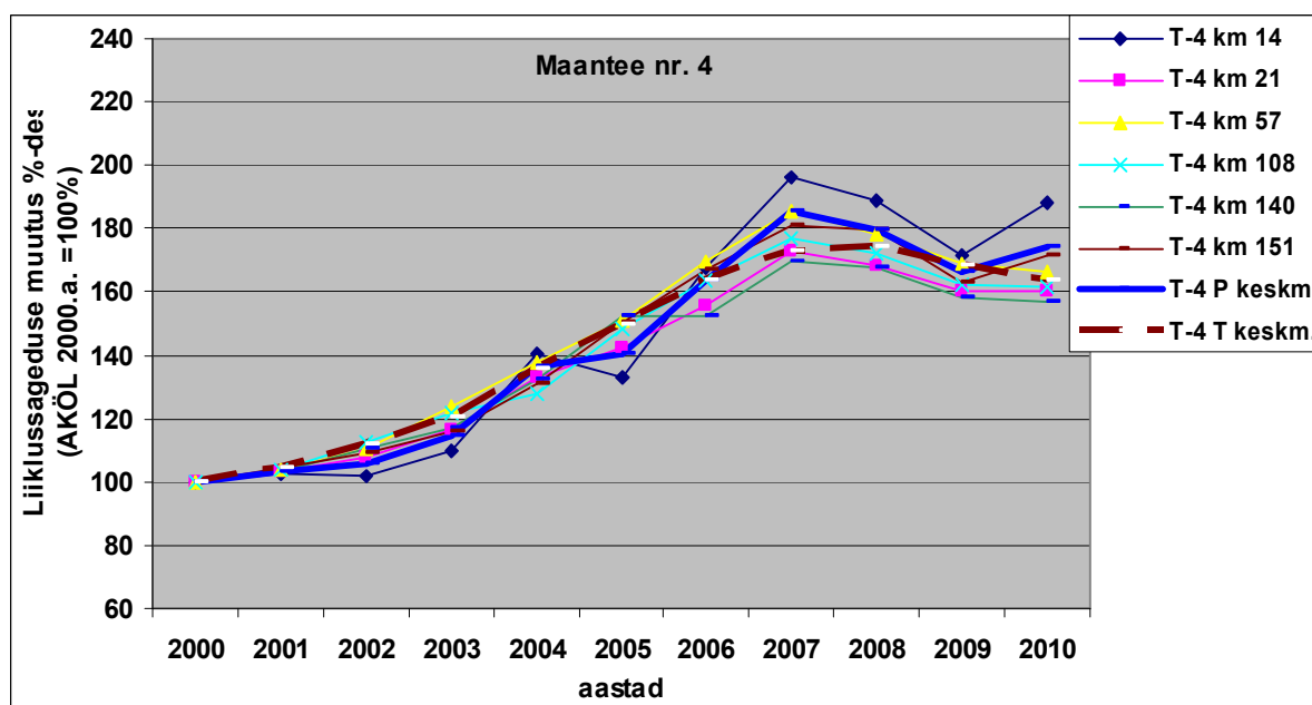
Joonis 1.7 Aasta keskmise ööpäevase liiklussageduse muutused Tallinn – Pärnu – Ikla maantee püsiloenduspunktides ja kogu maanteel keskmisena perioodil 2000 – 2010
