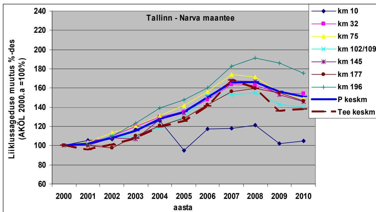
Joonis 1.4 Aasta keskmise ööpäevase liiklussageduse muutused Tallinn – Narva maantee püsiloenduspunktides ja kogu maanteel keskmisena perioodil 2000 – 2010
