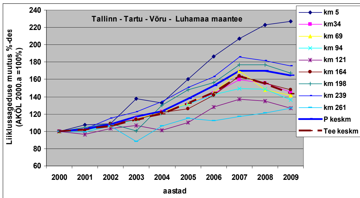
Joonis 1.5 Aasta keskmise ööpäevase liiklussageduse muutused Tallinn – Tartu – Võru – Luhamaa maantee püsiloenduspunktides ja kogu maanteel keskmisena perioodil 2000 – 2010
