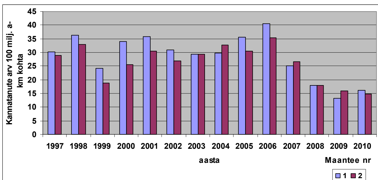
Joonis 3.9 Liiklusõnnetustes kannatanute (hukkunud ja vigastatud) absoluutarv, suhtearv maantee kilomeetri kohta ja maanteel sooritatud läbisõidu kohta Tallinn – Narva ja Tallinn – Tartu – Võru – Luhamaa maanteel aastatel 1997 – 2010
