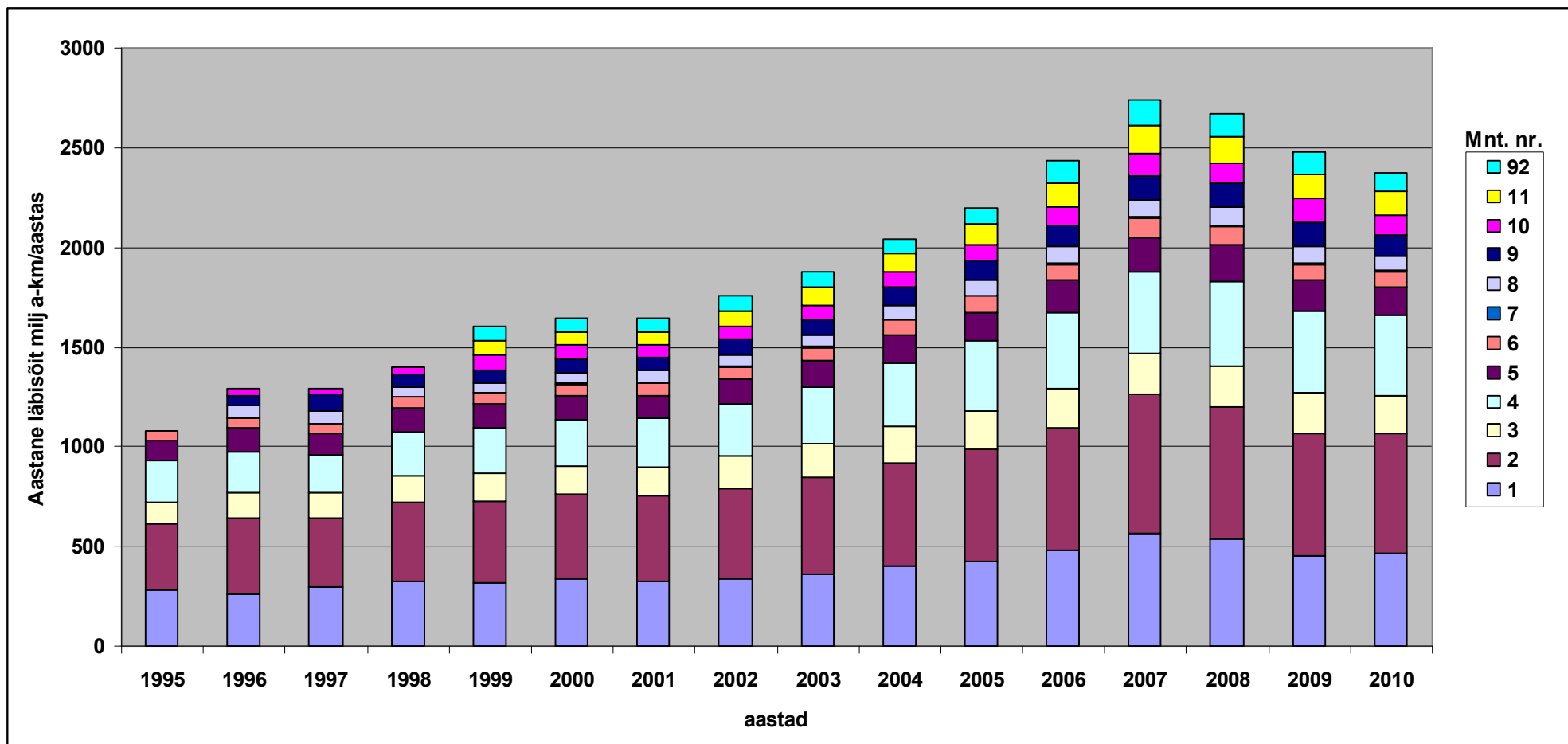
Joonis 1.11 Aastane läbisõit põhimaanteedel lõikes
