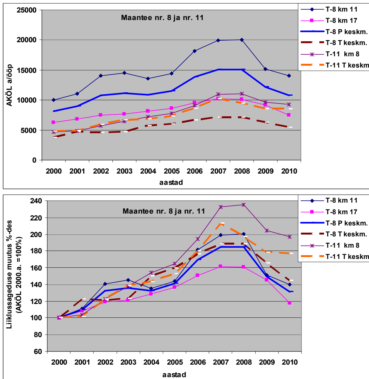
Joonis 1.9 Aasta keskmise ööpäevase liiklussageduse muutused Tallinn – Paldiski maantee ja Tallinna ringtee püsiloenduspunktides ning kogu maanteel keskmisena perioodil 2000 – 2010
