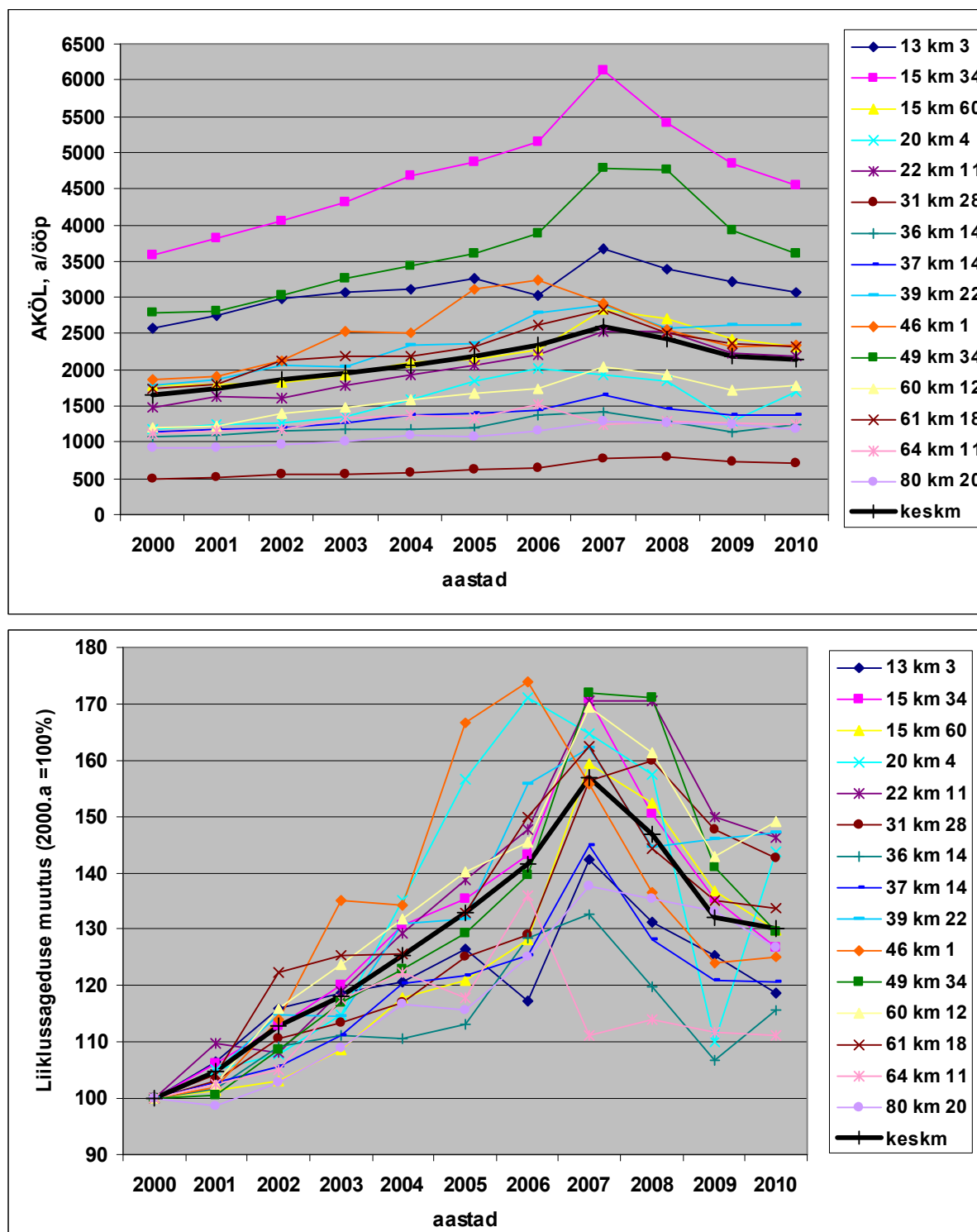
Joonis 1.19 Liiklussagedused ja nende muutus tugimaanteed püsiloenduspunktides aastatel 2000 - 2010
