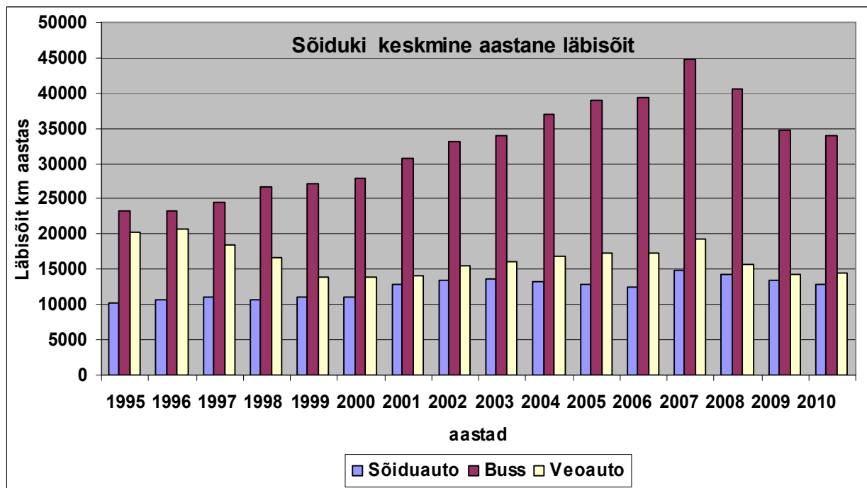
Joonis 1.36 Aasta keskmine läbisõit registris arvel oleva sõiduki kohta perioodil 1995 - 2010
