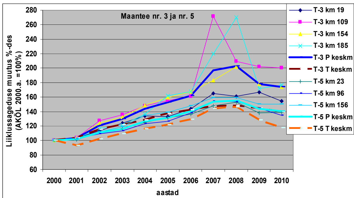
Joonis 1.6 Aasta keskmise ööpäevase liiklussageduse muutused Jõhvi – Tartu – Valga maantee ja Pärnu – Rakvere – Sõmeru püsiloenduspunktides ning kogu maanteel keskmisena perioodil 2000 – 2010
