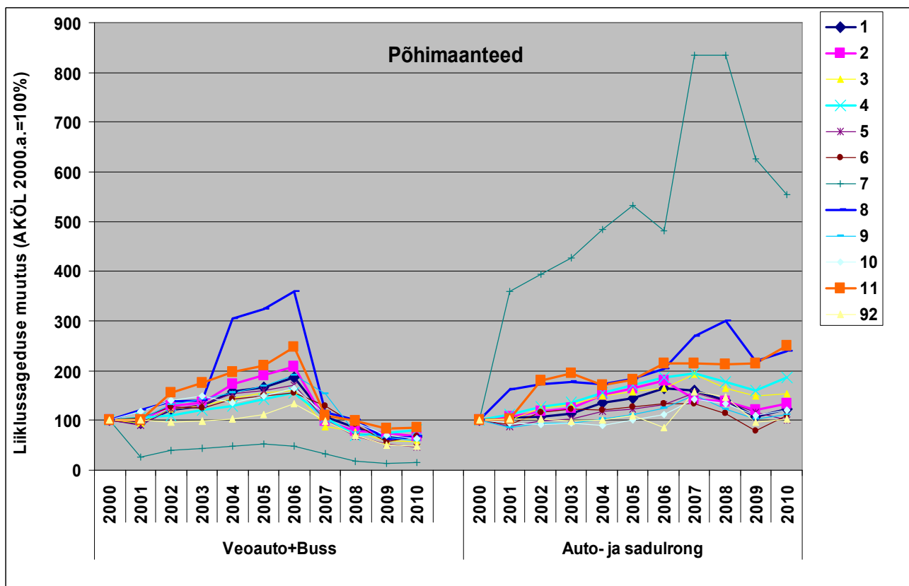
Joonis 1.14 Keskmise liiklussageduse muutus liikide lõikes aastatel 2000 - 2010
