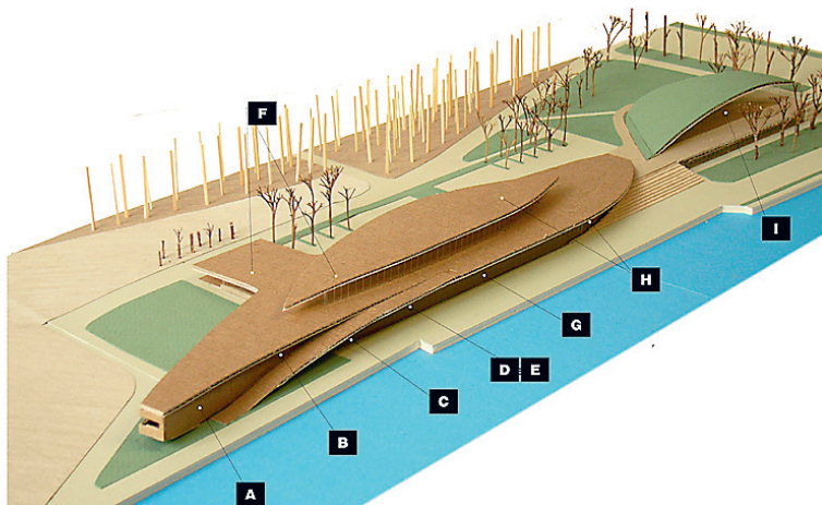
A vetelpäästjad, B ladu, C riietumisruumid, D surfikool, E surfiklubi, F kohvik, G sporditarvete kauplus, H spordiklubi, I suvesadam ja vabaajakeskus.
