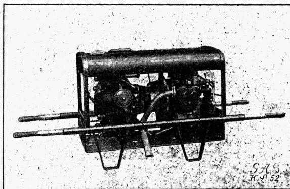
A.-S. Serlachiusse kantav mootorprits.
