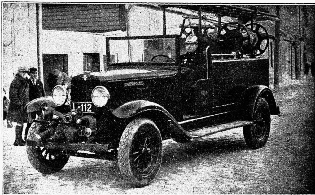
Haapsalu vabatahtliku tuletõrje ühingu autoprits, paagi mahutus 1560 l. Valmistatud Läänemaa tööstuskoolis 1931. a.
