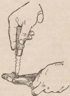
Рис. 55. Вывинчивание винта отсечки-отражателя
