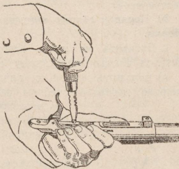
Рис. 54. Вывинчивание винта спусковой пружины
