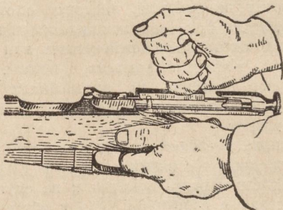
Рис. 46. Как вынуть затвор
