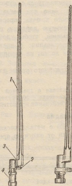
Рис. 26. Штык винтовки обр. 1891/30 г.:
