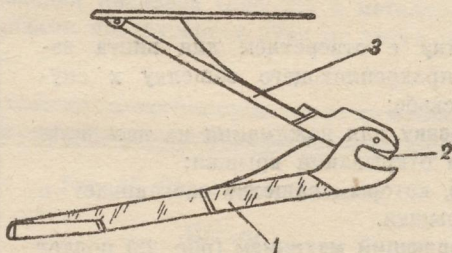
Рис. 22. Крышка магазинной коробки с подающим механизмом: 1—крышка, 2—вырез, 3—подающий механизм
