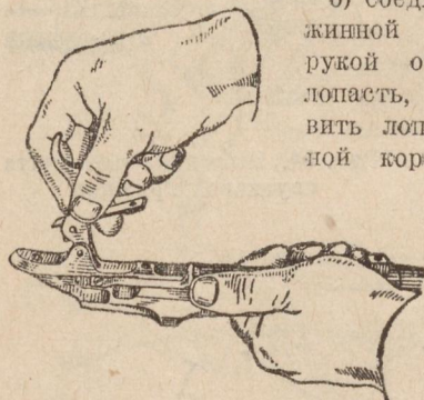
Рис. 56. Как вложить спусковой крючок со спусковой пружиной
