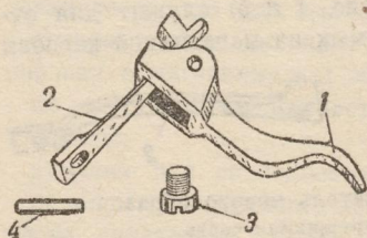
Рис. 6. Спусковой механизм: 1 — спусковой крючок, 2 — спусковая пружина, 3 — винт спусковой пружины, 4 — шпилька
