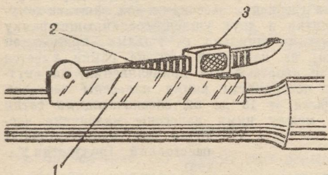
Рис. 7. Прицел винтовки обр. 1891/30 г.: 1 — прицельная колодка, 2 — прицельная планка, 3 — хомутик
