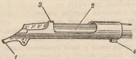
Рис. 3. Ствольная коробка:
