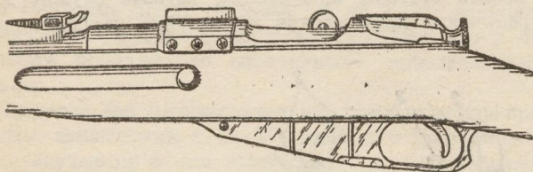
Рис. 95. Основание кронштейна, установленное на винтовке
