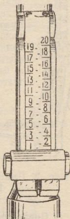
Рис. 8. Прицельная планка с хомутиком винтовки обр. 1891/30 г.
