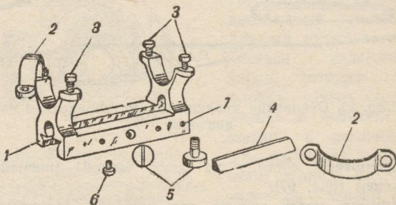
Рис. 97. Кронштейн:
