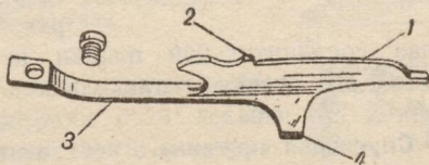
Рис. 5. Отсечка-отражатель старого образца:
