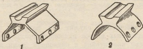
Рис. 96. Основание кронштейна: 1—для граневой ствольной коробки, 2—для круглой ствольной коробки
