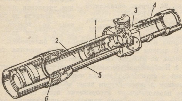
Рис. 93. Оптический прицел в разрезе:
