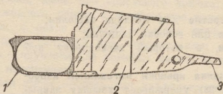
Рис. 21. Магази́нная коробка: 1—спусковая скоба, 2—щека, 3—угольник
