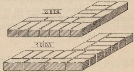
Joon. 5. Saviplonnidest poolteise kivi paksuse müüri ladumine.
