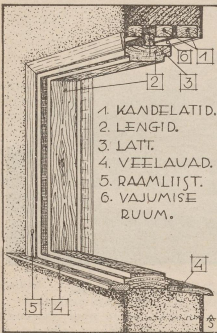
Joon. 14. Aken saviseinas.
