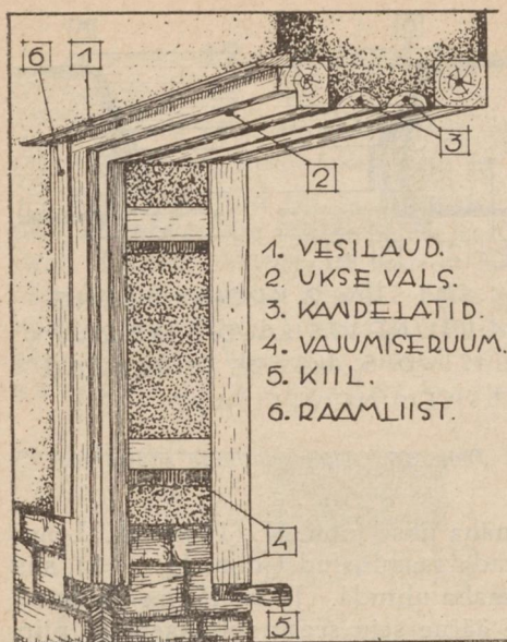
Joon. 17. Uks saviseinas.
