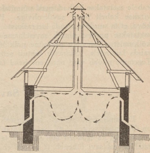
Joon. 9. Õhuvahetus läbi seina kanalite ja õhutoru.
