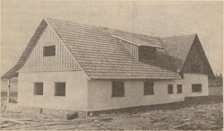
Savist koosehitus Tartumaal; seinad kaetud savikrohviga.
