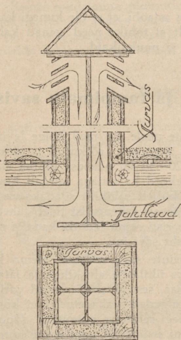
Joon. 8. Õhuvahetus neljaks jagatud õhutoru läbi.
