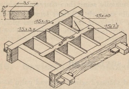
Joon. 4. Laudadest vorm saviplonnide tegemiseks.
