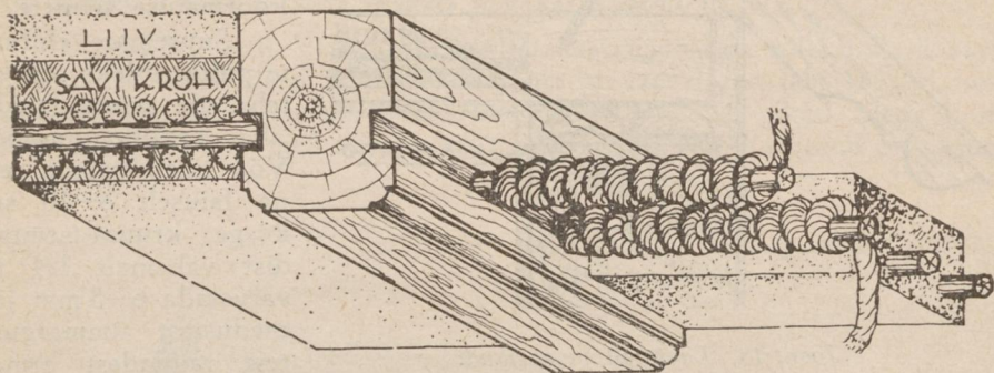
Joon. 12. Kaika-õlg savilagi.
