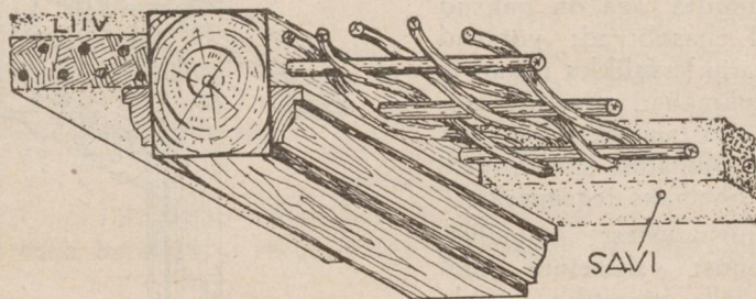
Joon. 11. Kaigastest ja vitsadest põimitud savilagi.
