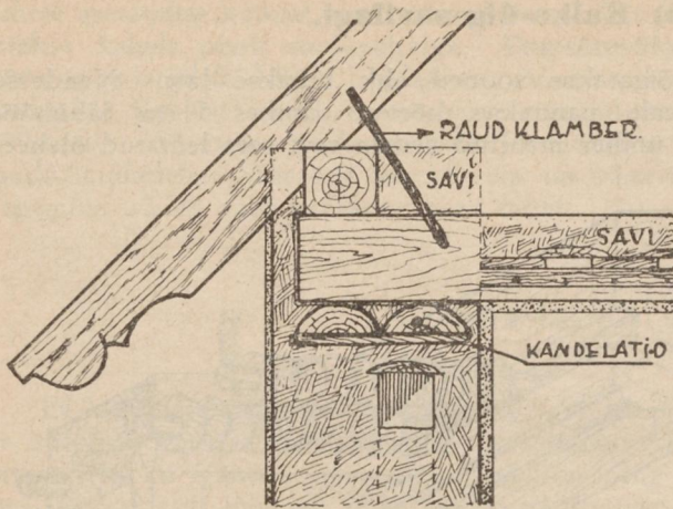
Joon. 13. Laetalad ja sarikad.
