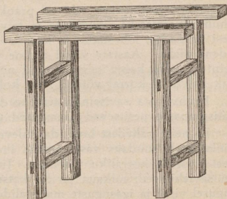
Joon. 16. Uste ja väravate piidad.
