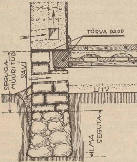
Joon. 1. Saviseina alusmüür.
