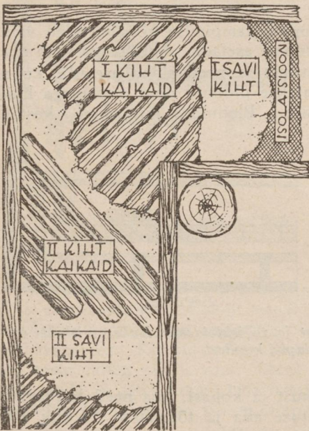
Joon. 7. Kaigastest saviseinte ladumine.
