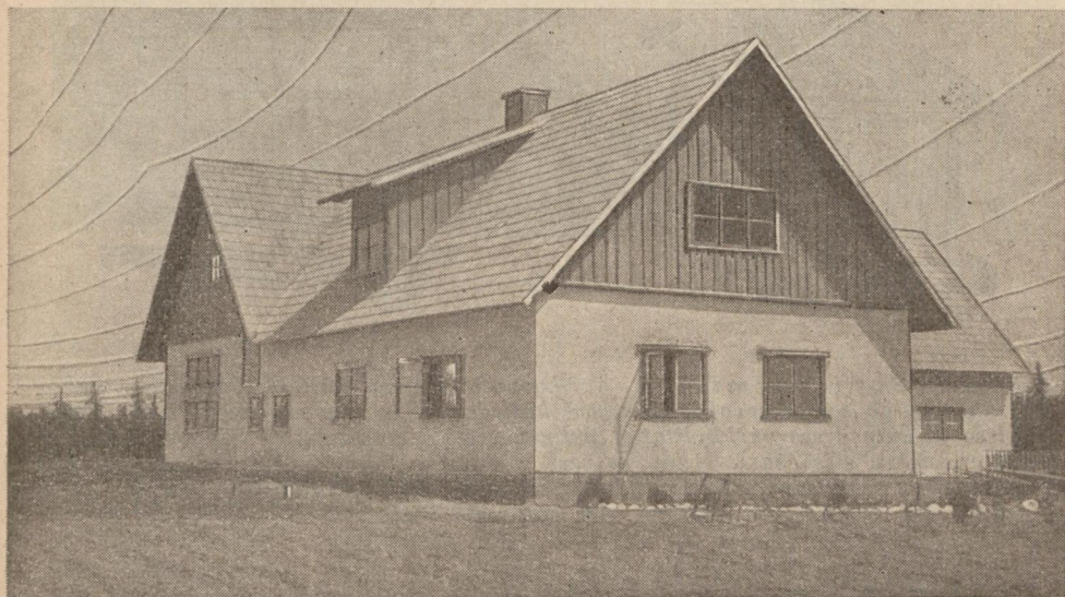
Asunduskomisjoni poolt ehitatud savist koosehitus, Tartumaal; seinad kaetud savikrohviga.
