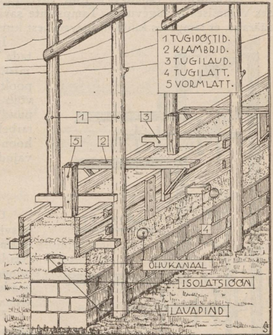
Joon. 2. Vormkastide vahele tambitud savisein.
