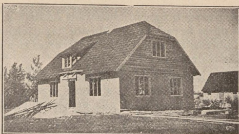
Savist elumaja ehitamisel.
