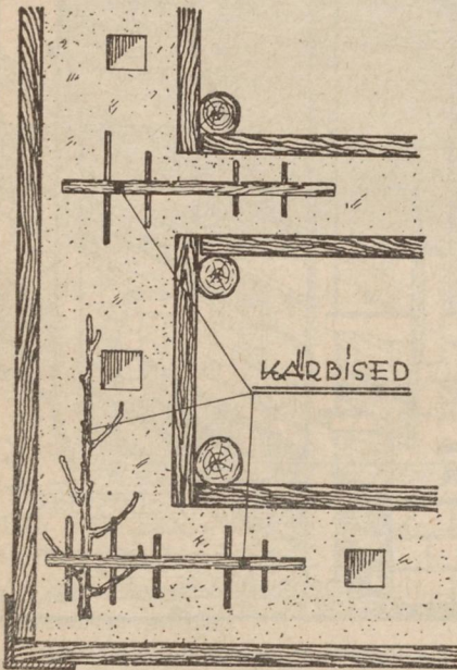
Joon. 3. Kärbised saviseinte nurkades ja vaheseintes.
