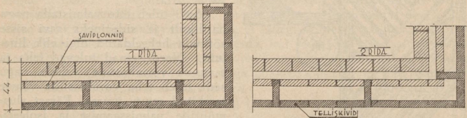
Joon. 6. Segaseina ladumine saviplonnidest ja telliskividest. Kaks väliskiht on serviti ja sisekiht lapiti kividest.
