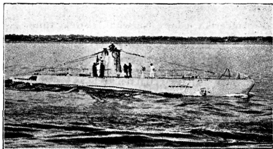
Saksa a-laev U-9. Elemendid: veeväljasurve 250 t., kiirus — \frac{13}{7} s.; relvastis — 1 rk ja 3 torp. Määratud tegevuseks Balti merel.
