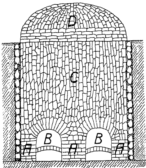
Täidetud lubjaahju esikülg. A — jalg, B — küttekolded, C — rind, D — keris.
