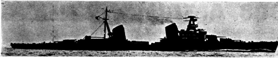
N. Vene uus ristleja „Kirov“. 8000 t.; kiirus 38 s., relvastus 9—180 mm suurt.; 4—76 mm õk-suurt.; 6—533 mm torpeedotoru
