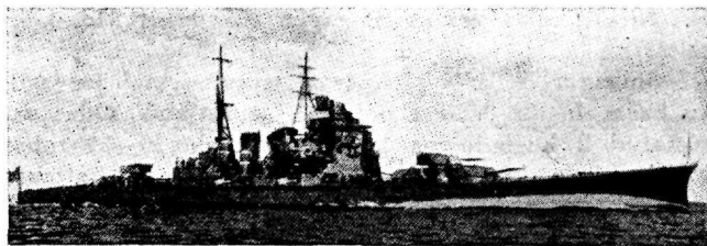
Jaapani ristleja „Atago“, 9850 t.; relvastus 10–20,3 sm, 8–12 sm 8–53,3 sm t.-t., 4 lennukit, 2 katapultit; kiirus 33 s.
