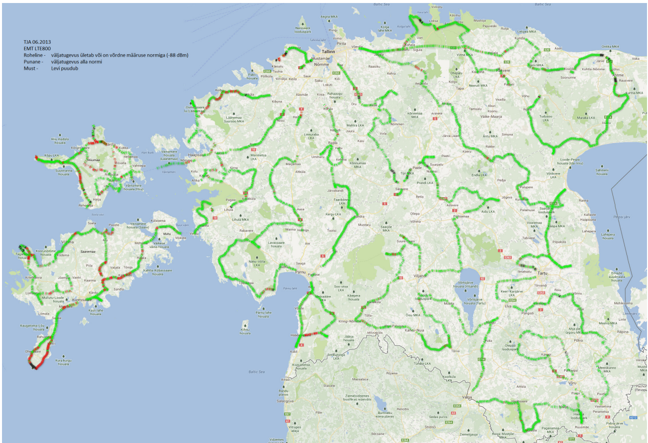
EMT 4G LTE 800 MHz võrgu katteala mõõtmise tulemus
