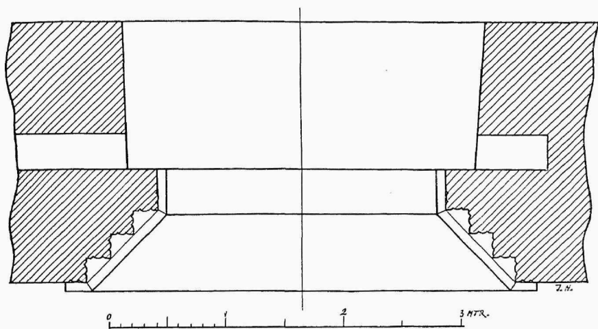
Läbilõige peaportaalist, joonistanud kunstnik J. Naha. — Huvudportalen, sektion. Ritad av konstnären J. Naha.
