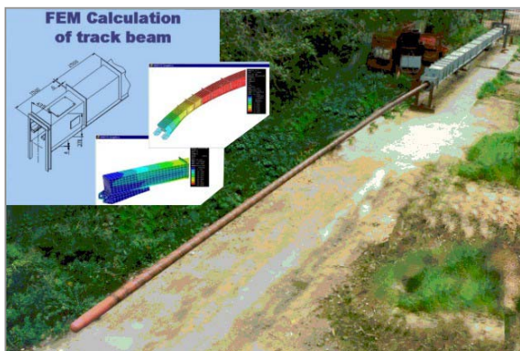
Joonis 3. 18m tahmapuhur.
