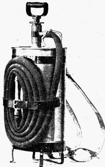
Seljaskantav hüdropult.
