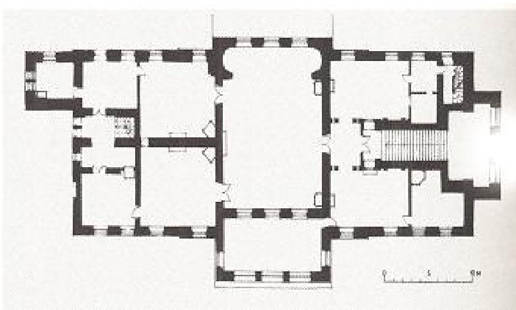
Muuga mõisa II korruse plaan Neff'ide ajal: 1860 – 1940.
